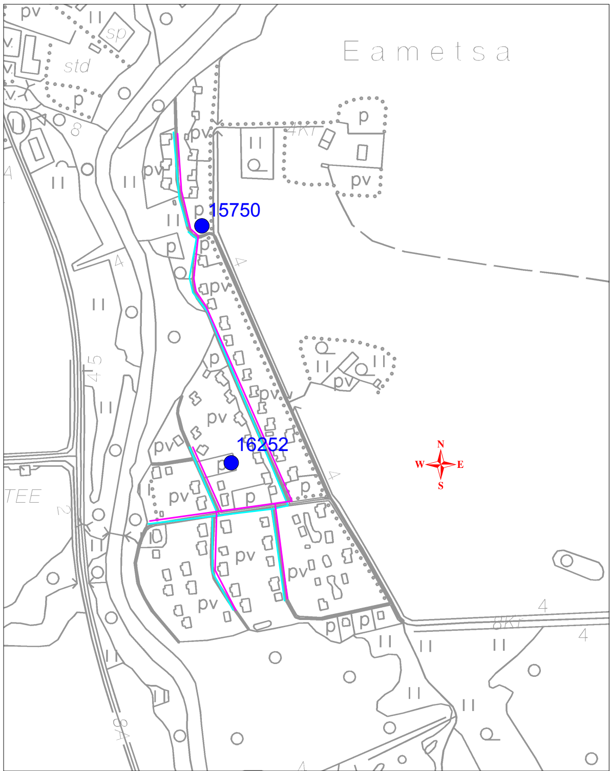
LISA 6B. Eametsa küla ühisveevarustuse ja kanalisatsiooni üldskeem
